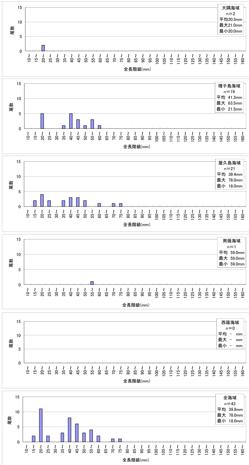
図1 採捕したモジャコの海域別全長組成(平成27年 3月調査)
