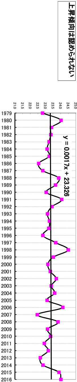
図 与路年平均水温の推移
