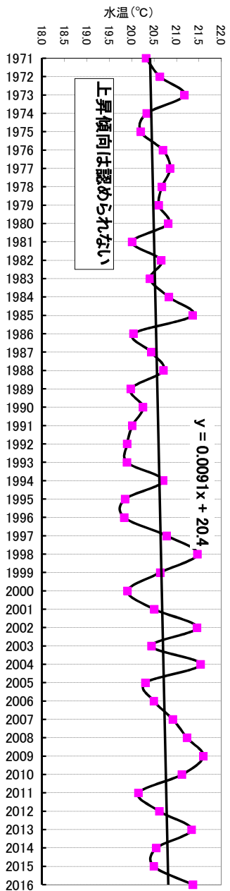
図 薩南沿岸年平均水温の推移 (代表点：竹島)
